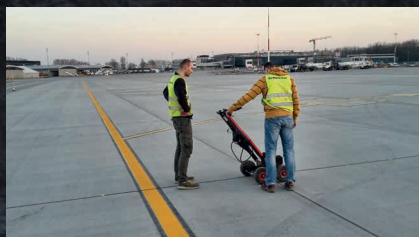
Port Lotniczy Kraków Balice – badania georadarowe nawierzchni drogi kołowania
