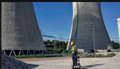
PGE Elektrownia Turów – badania georadarowe w rejonie budowy nowego bloku energetycznego
